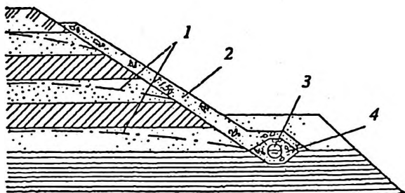
Рис. 31. Пластовый дренаж на откосах котлована: 1 - пониженные уровни подземных вод; 2 - песчаная пригрузка; 3 - дренажная труба; 4 - засыпка гравием
