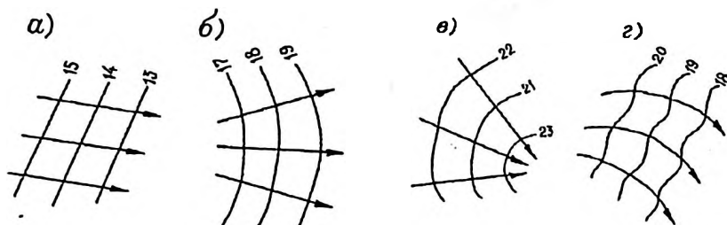
Рис.13. Потoki грунтовых вод: а) - плоский; б) – радиальный расходящийся; в) – радиальный сходящийся; г) – криволинейный
