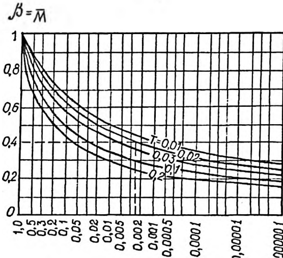
Рис.21. График для расчетов коэффициента несовершенства скважины \alpha .
