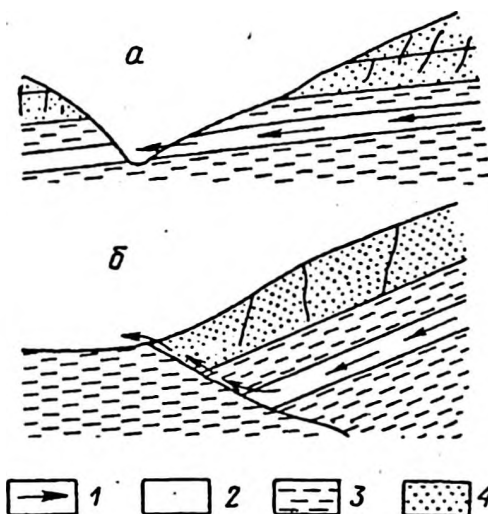
Рис. 10. Схема нисходящего (а) и восходящего (б) источников. 1 - направление движения воды и источники; 2 - водоносные породы; 3 - водоупорные породы; 4 - водопроницаемые породы.
