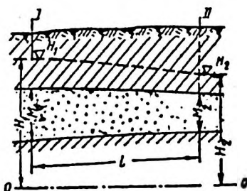
Схема напорного потока
