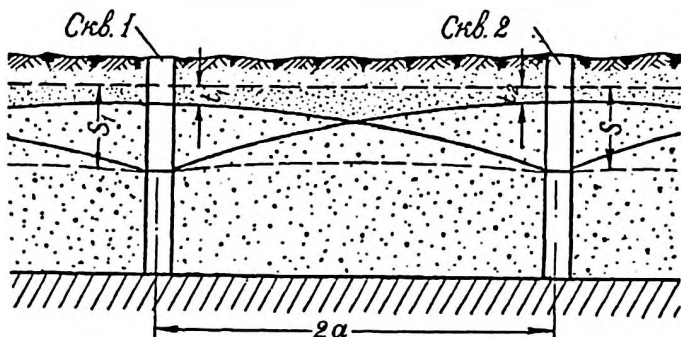
Рис. 25. Схема взаимодействия двух скважин
