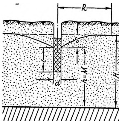
Рис. 23. Несовершенный грунтовый колодец
