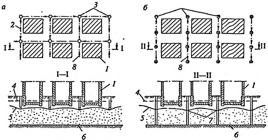
Рис. 30. Схема систематического дренажа: а - горизонтального; б - вертикального: 1 — контур защищаемого сооружения; 2 - ось горизонтального дренажа; 3 - смотровые колодцы; 4 - непониженный уровень грунтовых вод; 5 - пониженный уровень грунтовых вод; 6 - водоупор; 7 - вертикальные дрены; 8 - направление отвода дренажных вод
