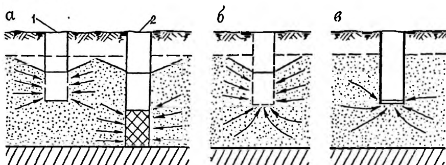
Рис.20. Типы несовершенных грунтовых колодцев:
