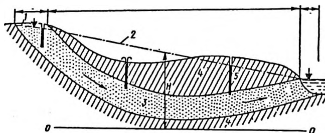
Рис. 7. Артезианский бассейн. Области: а - питания напорных вод; б - напора; в - разгрузки; 1 - уровень грунтовых вод; 2 - пьезометрический уровень напорных вод; 3 - водоносный напорный пласт; 4 - водоупоры; 5 - скважины; H - величина пьезометрического напора
