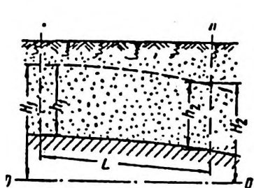
Схема грунтовых вод в наклонном пласте
