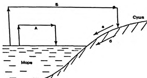
Рис. 1. Крутооборот воды в природе: А - малый; Б - большой; а - наземным путём; б - подземным путём
