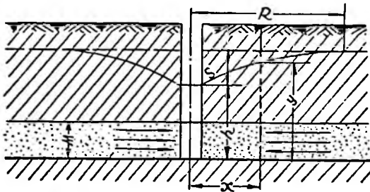
Рис. 19. Схема притока воды в артезианский колодец
