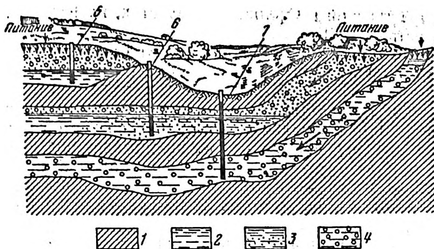
Рис. 3. Схема залегания подземных вод: 1- водоупорные породы; 2 - грунтовые воды; 3 - межпластовый безнапорный водоносный горизонт; 4 — артезианский напорный водоносный горизонт; 5 - колодец, питающийся грунтовой водой; 6 - колодец, питающийся межпластовой водой; 7 - артезианская скважина
