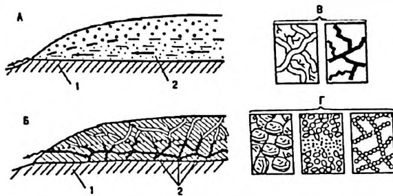
Рис. 2. А - пористые породы; Б - трещиноватые породы; В - размеры водопроводящих трещин; Г - размеры и плотность расположения зерен в пористых породах; 1 - водонепроницаемые породы; 2 - породы, насыщенные водой
