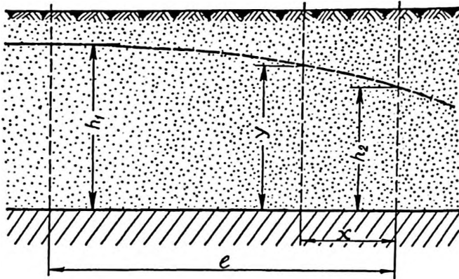
Рис. 15. Схема грунтового потока в горизонтальном пласте
