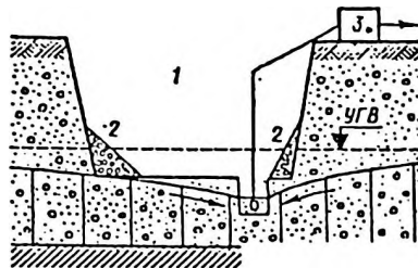
Рис. 28. Открытый водоотлив: 1 - котлован; 2 - пригрузка откосов; 3 - насос
