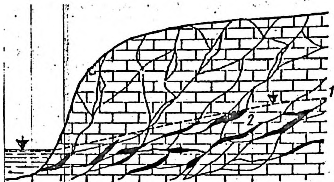
Рис. 9. Залегание карстовых вод в известняках: 1- уровень карстовых вод; 2 - зона карстовых пустот, заполненных водой
