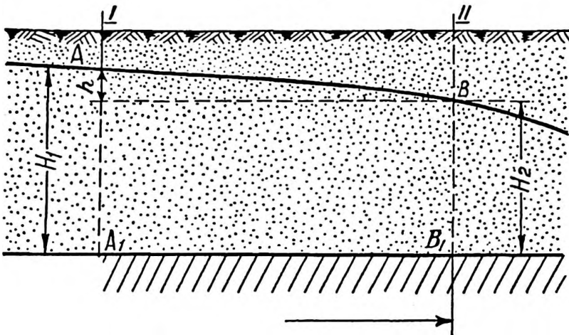
Рис. 14. Разрез участка подземного потока AB – уровень подземных вод; A 1 B 1 – водоупорное ложе; h – напор; l – длина пути фильтрации между сечениями I и II
