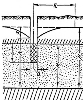
Рис. 22. Несовершенный артезианский колодец
