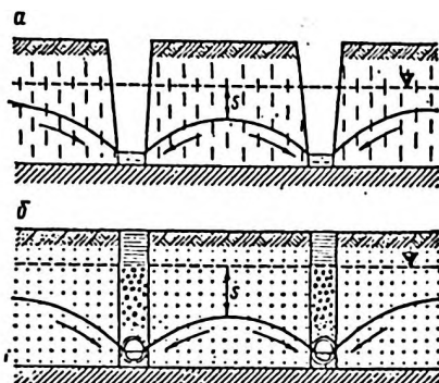
Рис. 27. Дренажные траншеи: а — открытые; б — закрытые
