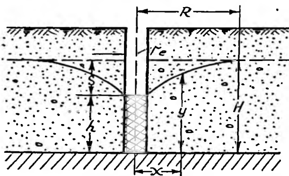
Рис. 18. Схема грунтового совершенного колодца
