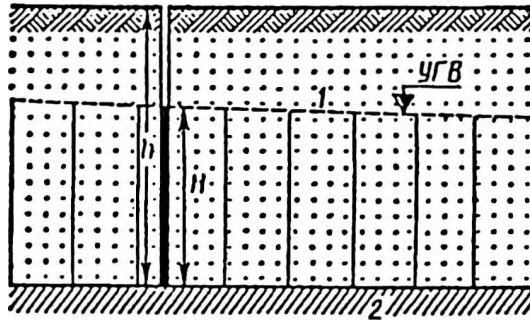
Рис. 5. Элементы грунтовой воды: h – мощность водопроницаемых пород; H – мощность водоносного горизонта; 1 – уровень грунтовой воды; 2 – водоупорное ложе
