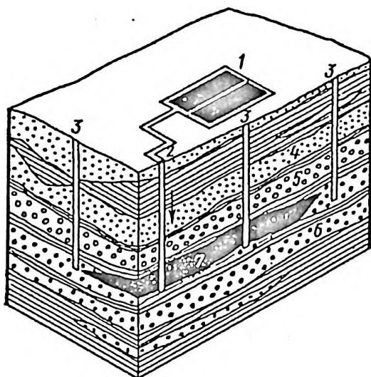
Рис. 33. Схема «захоронения» промышленных сточных вод в глубокие водоносные горизонты (по Н.В. Тарасовой):
