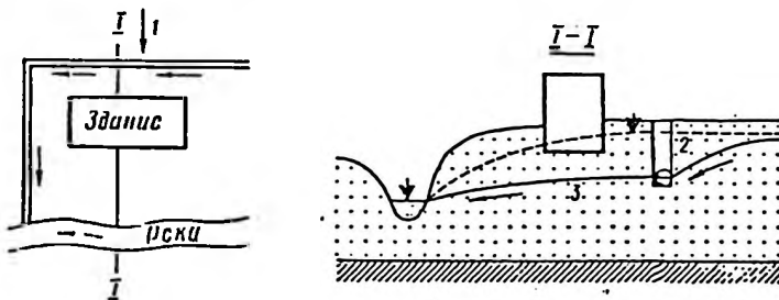
Рис. 29. Головной дренаж (план и разрез): I — направление потока грунтовых вод; 2 — головная дрена; 5 — сниженный уровень грунтовых вод
