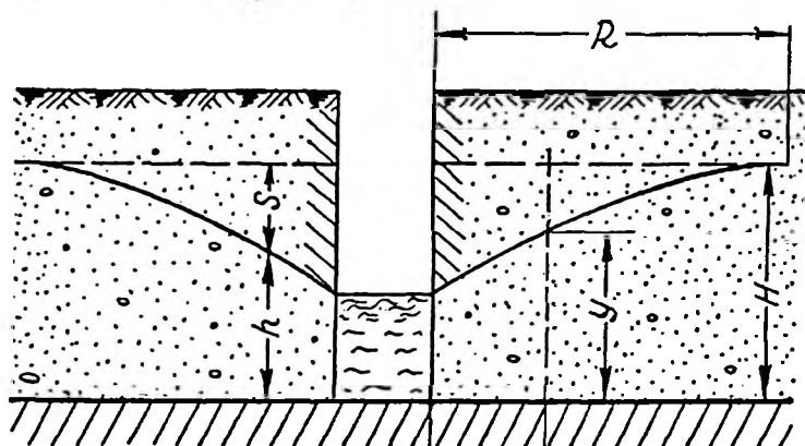
Рис. 24. Горизонтальная канава, доведенная до водоупора
