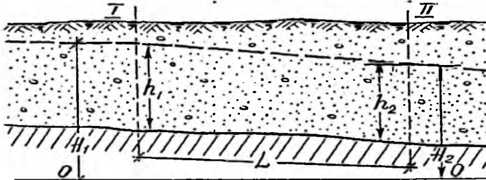
Рис. 16. Схема грунтовых вод в наклонном пласте
