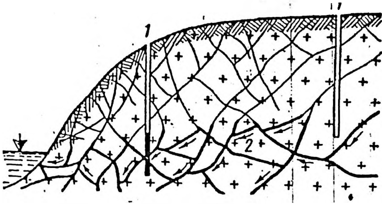
Рис. 8. Залегание трещинно-грунтовых вод: 1 - скважины; 2 - трещины с водой
