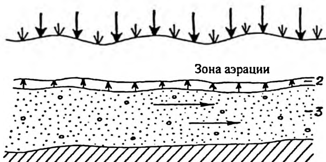
Рис. 4. Распределение подземных вод в верхней части земной коры: 1 — зона аэрации; 2- зона капиллярной воды; 3 — зона полного насыщения (грунтовый поток)
