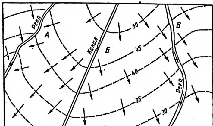
Рис. 6. Карта гидроизогипс: участок А - грунтовые воды питают реку; В - канал питает грунтовые воды; В - грунтовые воды питают реку и выходят из нее
