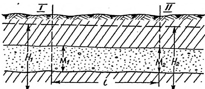
Рис. 17. Схема напорного потока
