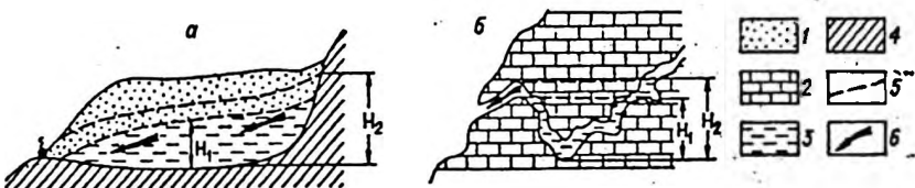
Рис. 11. Периодически действующие переливающиеся источники.
