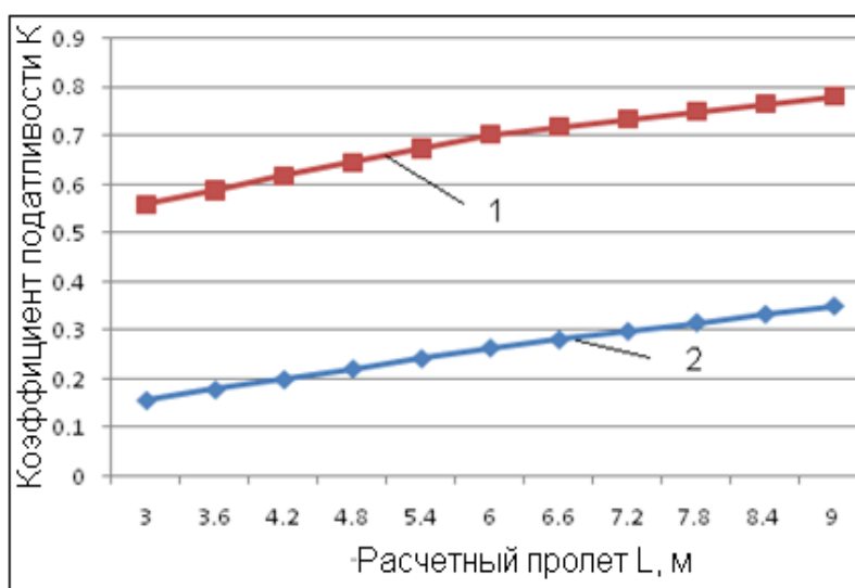
Рис. 1. Коэффициент податливости узлов заделки в стены плит с высотой сечения 220 мм, при коэффициенте \nu=0,5 (жилые и административные здания) для кладки без армирования сетками (1) и для кладки, армированной сетками (2)
