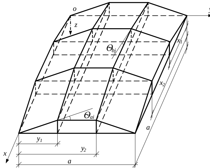
Рис. 2. Оболочка с изломами срединной поверхности в двух направлениях
