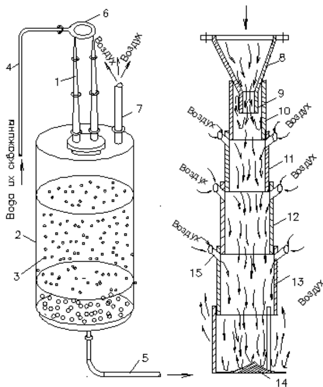
Рис.1. Вакуумно-эжекционная установка:
