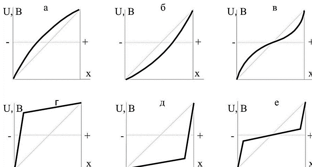
Рис. 1- Некоторые возможные варианты распределения потенциала в диэлектриках при высоковольтной поляризации
