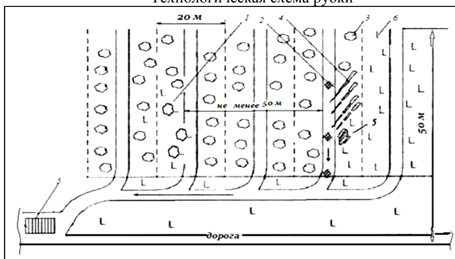
Рис. 6. Схема разработки лесосек бензиномоторной пилой и трелёвке форвардером: 1 – полупасека; 2 – * трелёвочный волок; 3 – растущий лес; 4 – поваленные деревья; 5 – Сортименты; 6 – L – вырубка; – направление трелёвки
