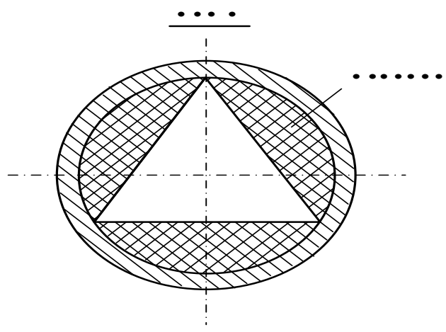
Рисунок 5 – Узел прессования с фильерой в виде треугольника
