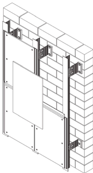
Рисунок 1 – Навесная вентилируемая фасадная система
