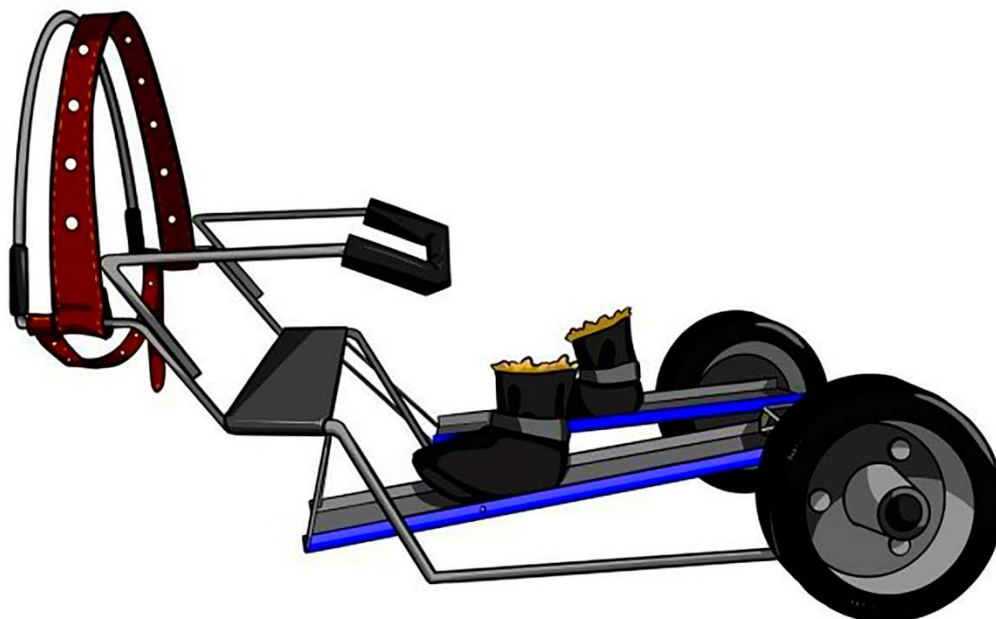
Рисунок 1 – Общий вид конструкции ходунков для собак с парезом бедренного нерва
