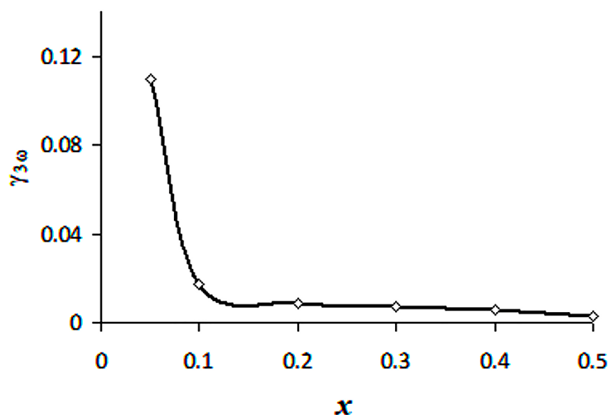
Рисунок 2 – Зависимости амплитуды \gamma_{3\omega} от процентного содержания нитрата рубидия в (\text{RbNO}_3)_x/(\text{KNO}_3)_{(1-x)}
