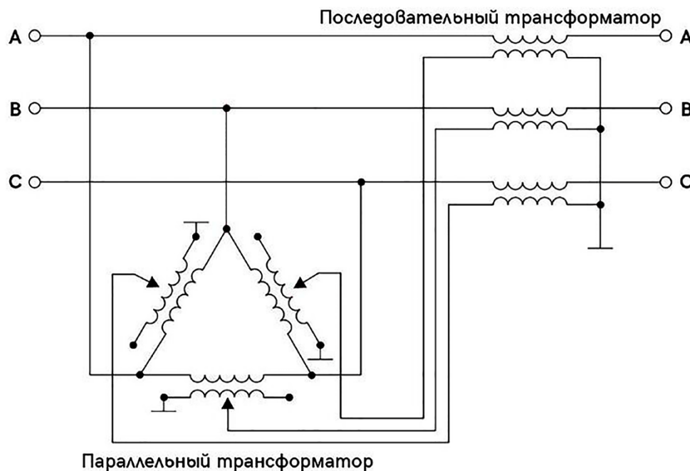
Рисунок 1 – Схема фазоповоротного трансформатора
