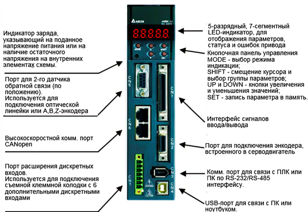
Рисунок 2 – Сервопреобразователь Delta ASD-A20421
