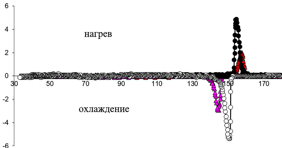
Рисунок 1 – Сигналы для объёмного (круги) и нанокомпозитного (треугольники) нитрата цезия
