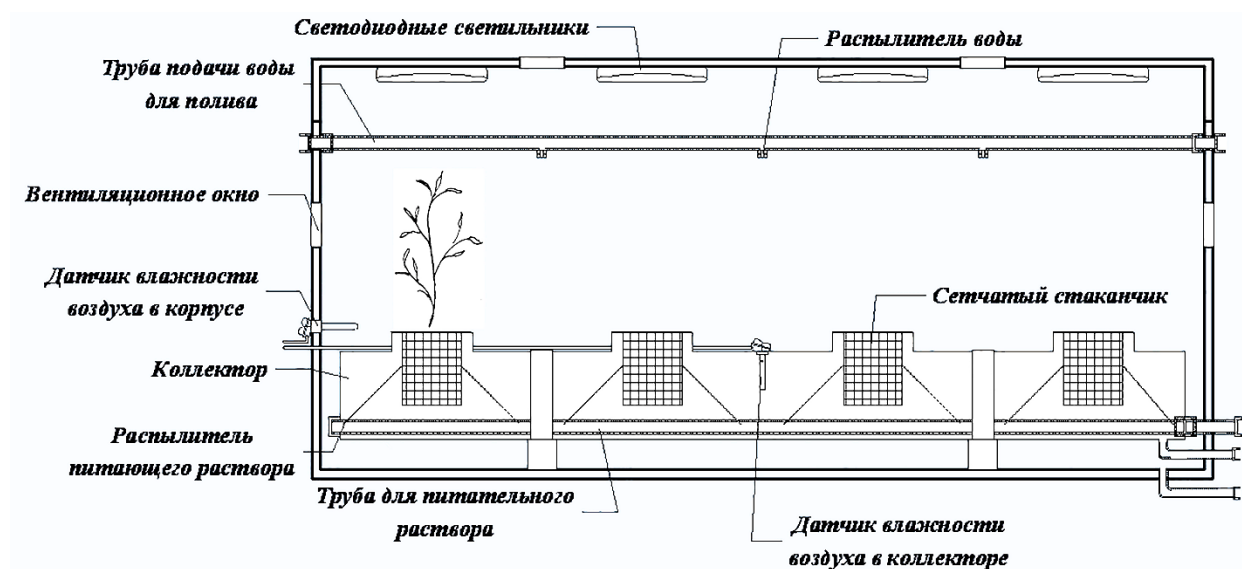
Рисунок 1 – Конструкция аэропонной установки
