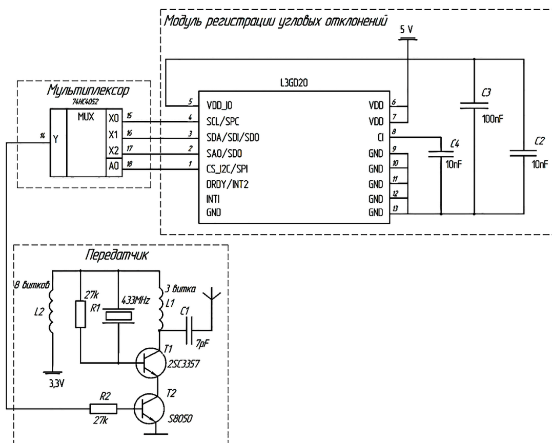
Рисунок 2 – Принципиальная схема калибровочного устройства
