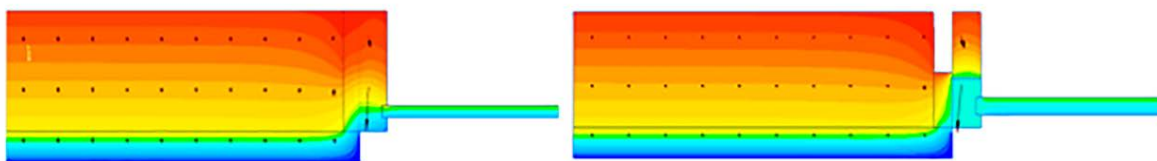
Рисунок 2 – Сечение с утеплителем 50 мм без дефекта и с дефектом монтажной пены. Расчёт графиков тепловых полей
