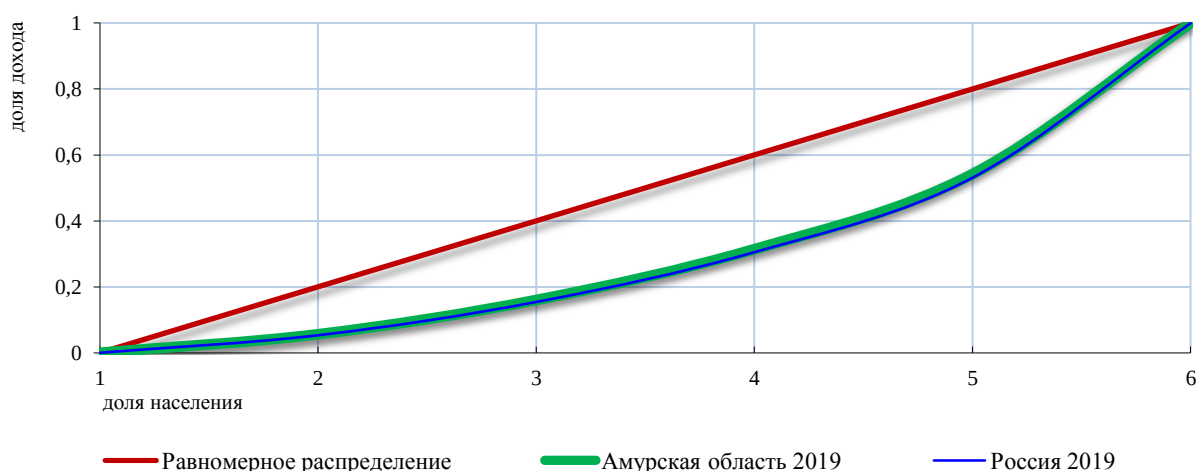
Кривая Лоренца
