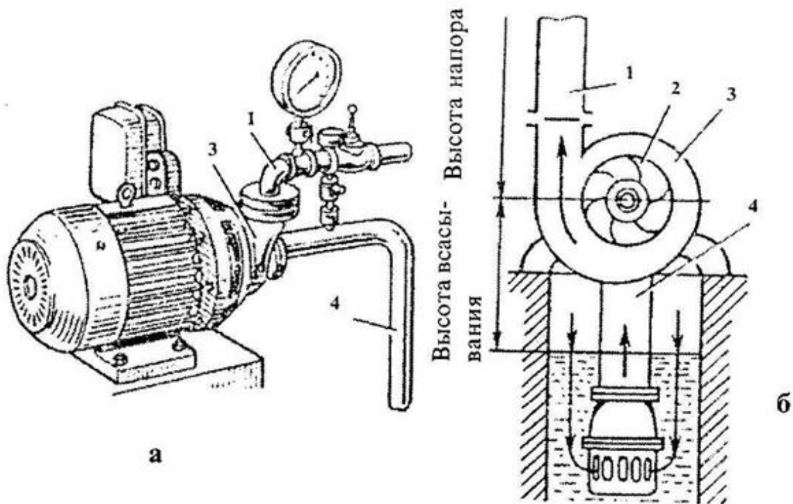
Рис. 1. Центробежный водяной насос: а – общий вид насоса с электродвигателем; б – схема насоса; 1 – нагнетательный трубопровод; 2 – рабочее колесо; 3 – корпус; 4 – всасывающий трубопровод.
