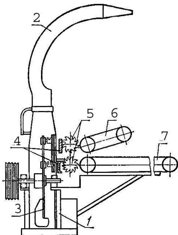
Рис. 5. Соломосилосорезка РСС-6,0Б: 1– рама; 2– дефлектор с поворотным устройством; 3– режущевыбросной аппарат; 4– гребёнки; 5 – прессующие валики; 6 – подпрессовывающий транспортёр; 7– подающий транспортёр.
