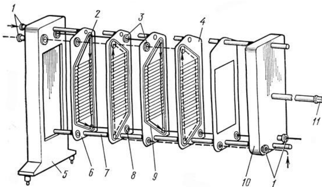
Рис. 25. Схема пластинчатого охладителя: 1 - штуцера, 2 - верхнее отверстие, 3 - кольцевые резиновые прокладки штанга, 8 - нижнее отверстие, 9 - большая резиновая прокладка 10 - зажимная плита, 11 - винт
