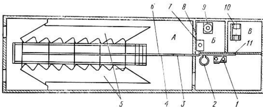
Рис. 23. Примерная планировка помещений доильной установки «Елочка» УДЕ-8: А - доильное отделение, Б - моечное отделение, В - вакуум-насосная; 1 - молочный насос, 2 - охладитель, 3 - молокопровод с фильтром, 4 - вакуум-провод, 5 - доильные станки, 6 - водяная магистраль, 7 - бак-смеситель, 8 - ручной насос, 9 - водогрейный котел, 10 - силовой агрегат, 11 - вакуум-баллон
