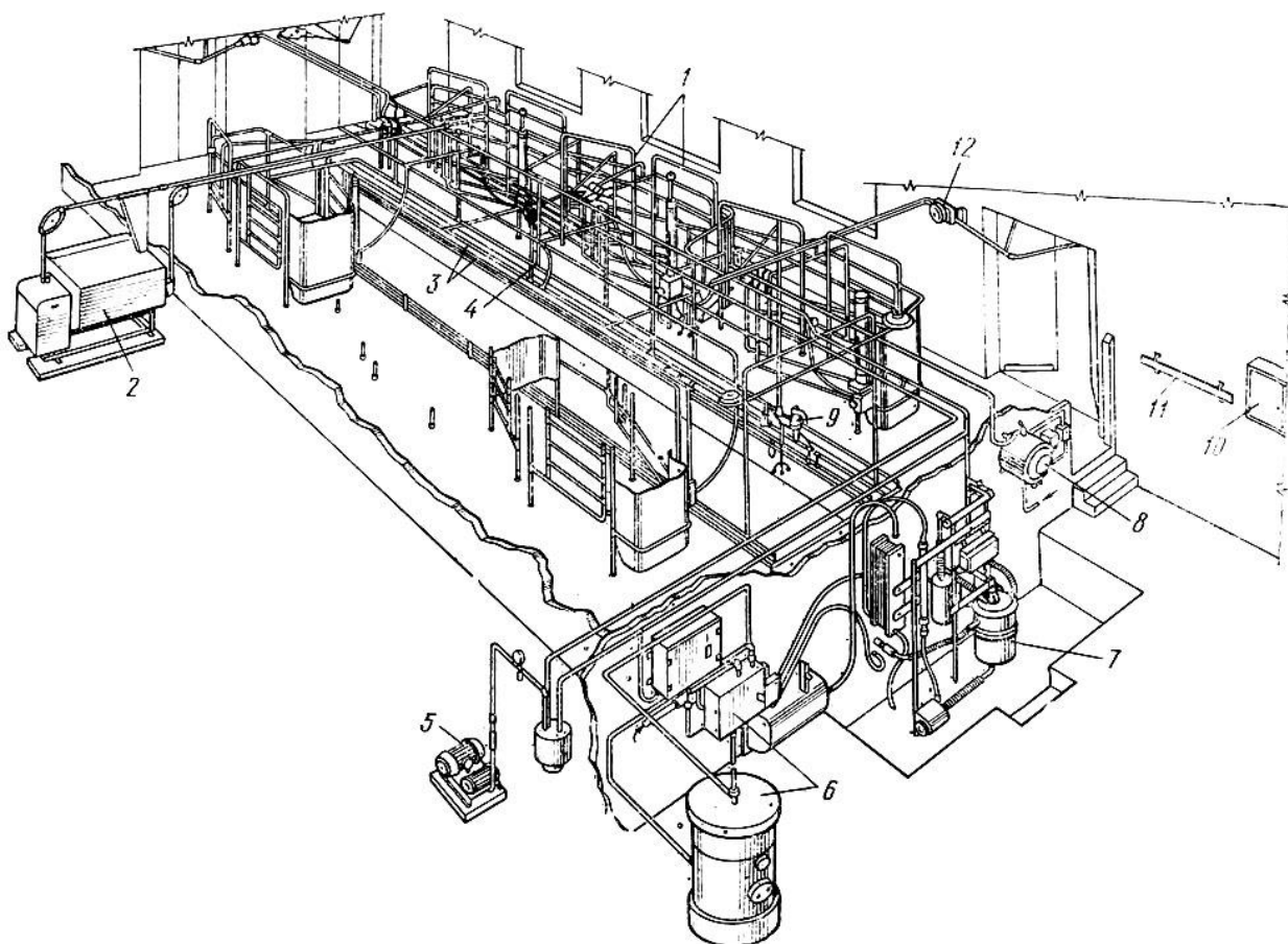
Рис. 23. Доильная установка 'Тандем' УДТ-6: 1 - доильные станки, 2 - система раздачи кормов, 3 - молокопровод, 4 - устройство для подмывания вымени, 5 - вакуумный насос, 6 - система промывки, 7 - охладитель, 8 - водонагреватель, 9 - доильные аппараты со счетчиками, 10 - шкаф для резиновых деталей, 11 - полка для счетчиков молока, 12 - пневмопривод дверей доильной площадки
