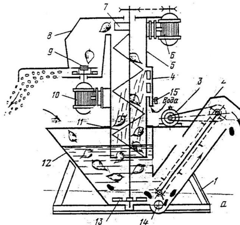
Рис. 3. Схема и общий вид измельчителя-камнеуловителя ИКМ-5 1—рама; 2—транспортёр-камнеудалитель; 3,6,10—электродвигатели; 4—гребёнка подвода воды; 5—кожух шнековой мойки; 7—выбрасыватель; 8—крышка измельчителя; 9—измельчитель;
