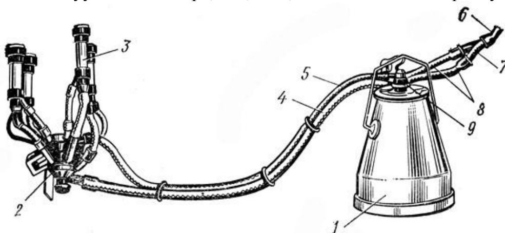
Рис. 18. Доильный аппарат ДА-2М «Майга»: 1 - ведро, 2 - коллектор, 3 - стаканы, 4 - молочный шланг, 5 - шланг переменного вакуума, 6 - шланг магистральный, 7 - тройник, 8 - шланги переменного вакуума, 9 - крышка ведра
