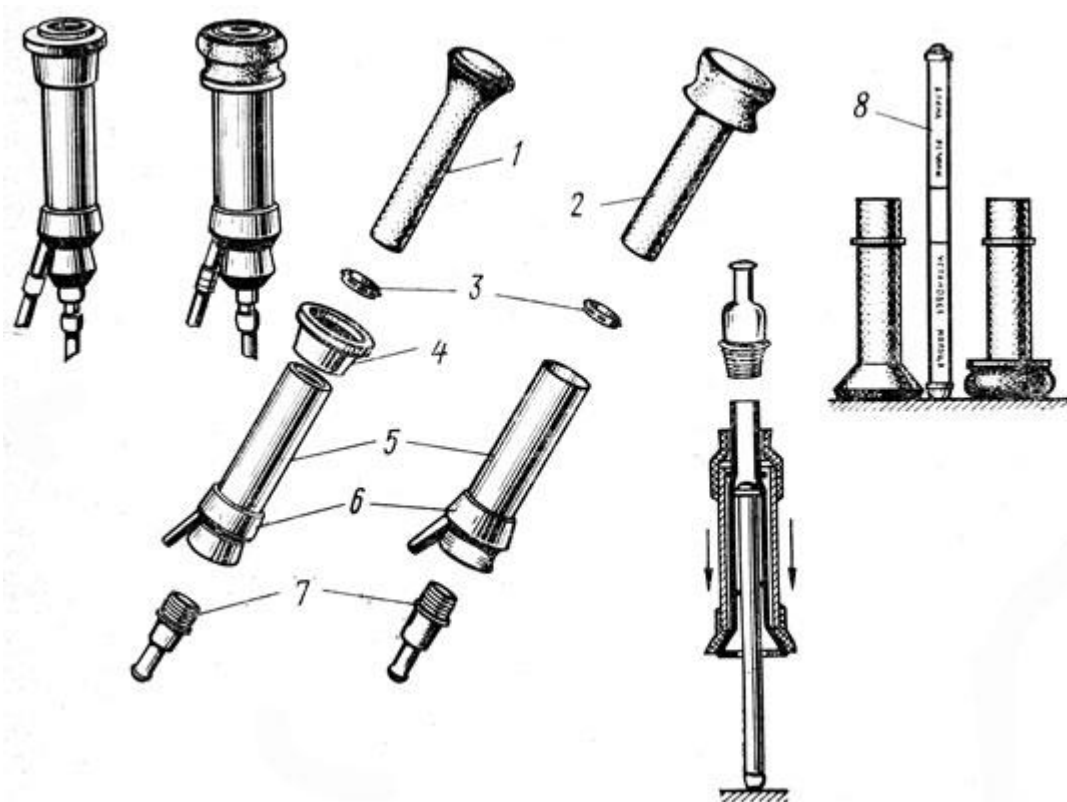
Рис. 21. Устройство и сборка доильного стакана: 1 и 2 - сосковая резина, 3 - монтажное кольцо, 4 - верхняя головка, 5 - гильза стакана 6 - нижняя головка, 7 - смотровой конус, 8 - монтажный стержень
