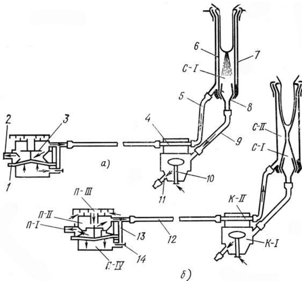
Рис. 17. Схема работы доильного аппарата ДА-2М 'Майга': а - такт сосания, б - такт сжатия; 1 - мембрана пульсатора, 2, 4, 13 - патрубков, 3, 10 - клапан, 5 - воздушный шланг, б - сосковая резина, 7 - гильза стакана, 8 - смотровой конус стакана, 9 - молочный шланг, 11 - молочный патрубок 12 - воздушный шланг, 14 - регулировочный винт, С-I и С-II - подсосковое и межстенное пространства стакана, К-I и К-II - камеры постоянного и переменного вакуума коллектора, П-I, П-II, П-III и П-IV - камеры пульсатора
