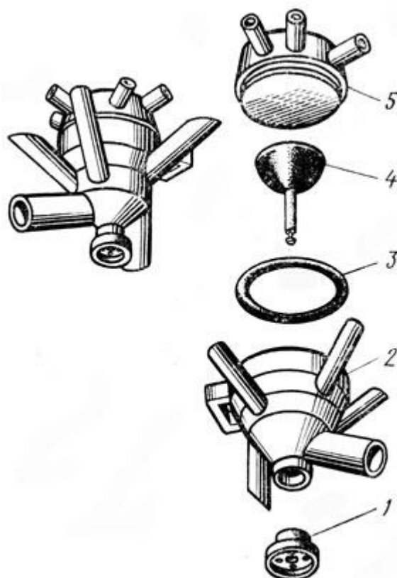
Рис. 20. Коллектор доильного аппарата ДА-2М «Майга»: 1 - шайба, 2 - корпус, 3 - прокладка, 4 - клапан, 5 - распределитель переменного вакуума
