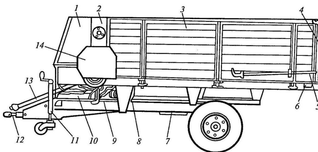
Рис. 13. Малогабаритный кормораздатчик РММ – Ф – 6: 1 – ограждение битеров; 2 – блок битеров; 3,4 – борта; 5- тяга; 6 и 10 – продольный и поперечный транспортёры; 7 – система пневмотормозов; 8 – редуктор; 9 – храповый механизм; 11 – домкрат; 12 – прицепная серьга; 13 – карданный вал; 14 - ограждение
