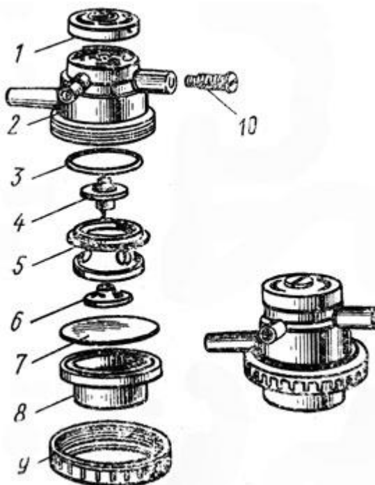
Рис. 19. Пульсатор доильного аппарата ДА-2М 'Майга': 1 - крышка, 2 - корпус, 3 - прокладка, 4 - клапан, 5 - диффузор, 6 - шайба, 7 - мембрана, 8 - корпус камеры, 9 - гайка, 10 - регулировочный винт
