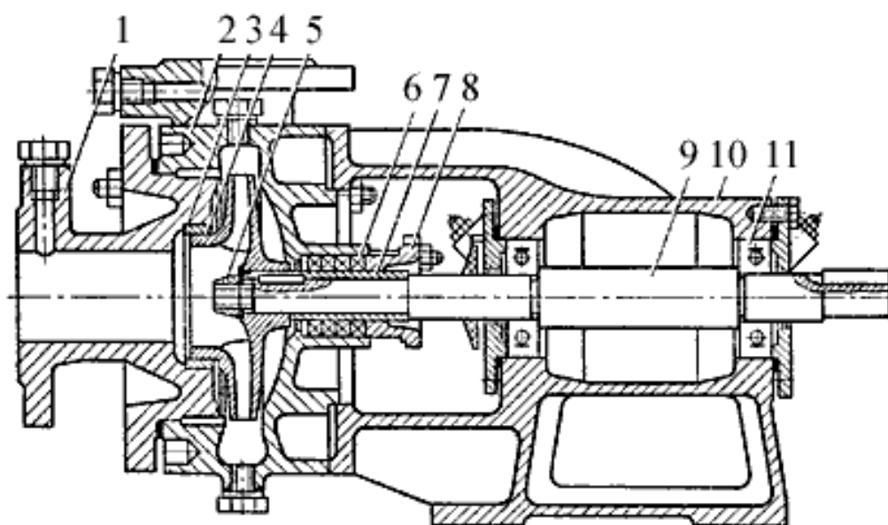
Рис.2. Устройство консольного насоса одностороннего всасывания типа К
