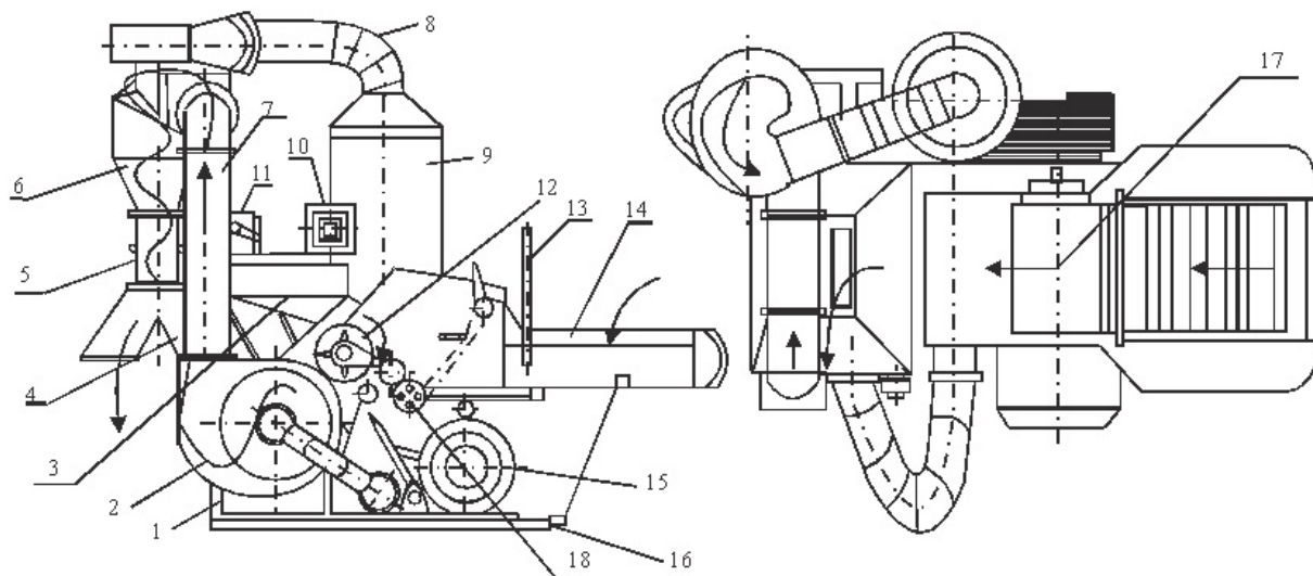
Рис. 9. Молотковая дробилка КДМ – 2 1 - дробильный аппарат; 2 - вентилятор; 3 - загрузочный бункер; 4 - рукав выгрузки; 5 - шлюзовой затвор; 6 - циклон; 7 - кормовой трубопровод; 8 - воздушный трубопровод; 9 - фильтрованный рукав; 10 - амперметр-индикатор; 11 - червячный редуктор; 12 - барабан ножевой; 13 рычаг включения; 14, 17 - подающий и прессующий транспортеры; 15 - электродвигатель; 16 - рама; 18 - редуктор
