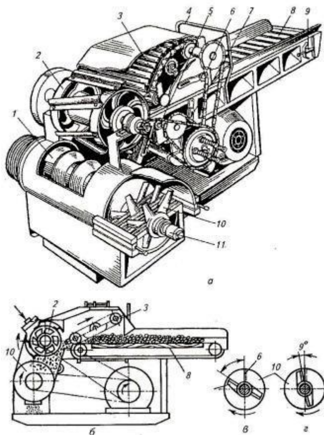
Рис. 4. Измельчитель кормов ИКВ-5А «Волгарь-5»
