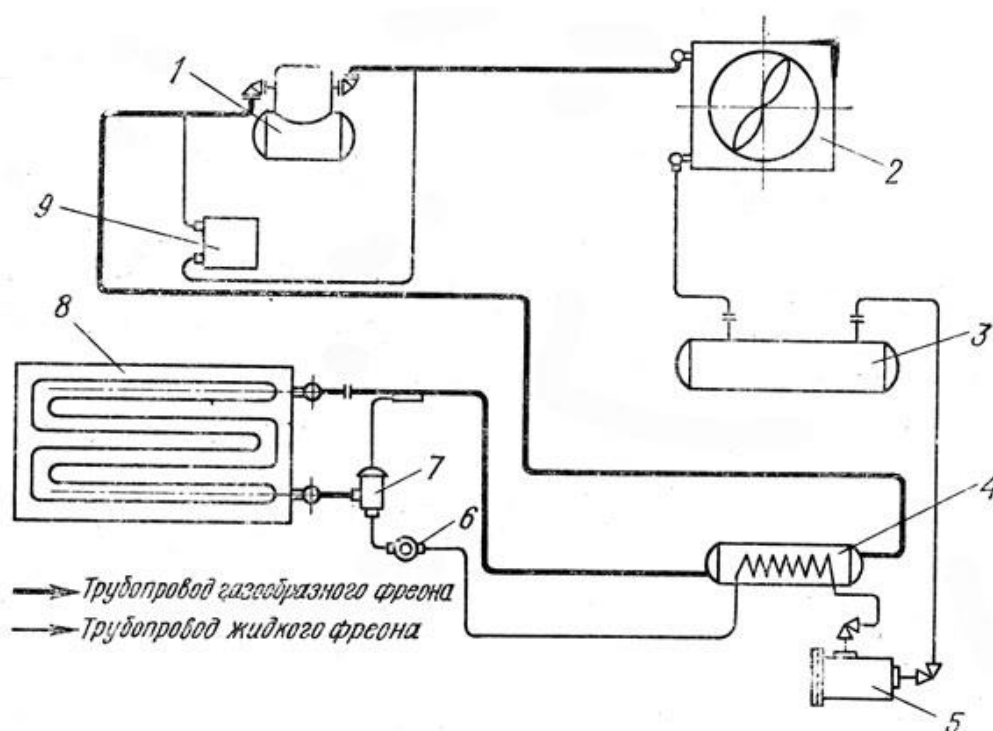
Рис. 24. Схема фреоновой холодильной установки МХУ-8: 1 - компрессор, 2 - конденсатор, 3 - ресивер, 4 - теплообменник, 5 - фильтр-осушитель, 6 - смотровое устройство, 7 - вентиль, 8 - испаритель, 9 - реле давления
