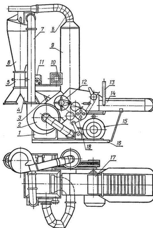
Рис. 8. Универсальная дробилка кормов КДУ-2,0: 1 – дробильный аппарат; 2 – вентилятор; 3 – загрузочный ковш; 4 – рукава выгрузки; 5 – шлюзовой затвор; 6 – циклон; 7 – кормовой трубопровод; 8 – воздушный трубопровод; 9 – фильтровальный рукав; 10 – амперметр –индикатор; 11 – червячный редуктор; 12 – ножевой барабан; 13 – рычаг включения; 14 – питающий транспортёр; 15 – электродвигатель; 16 – рама; 17 – подпрессовывающий транспортёр; 18 - редуктор
